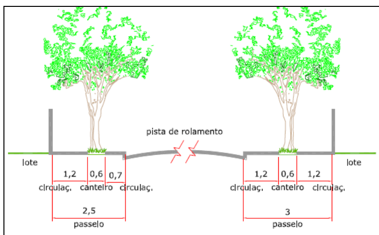
Figura 5 – Passeio ecológico. Fonte: MB Consultoria.
