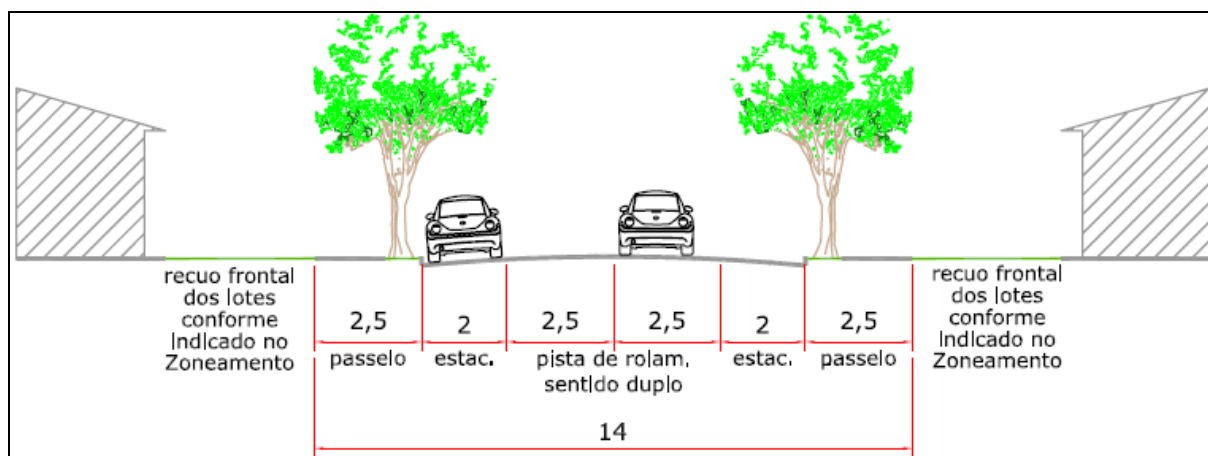
Figura 4 – Via Local. Fonte: MB Consultoria.
