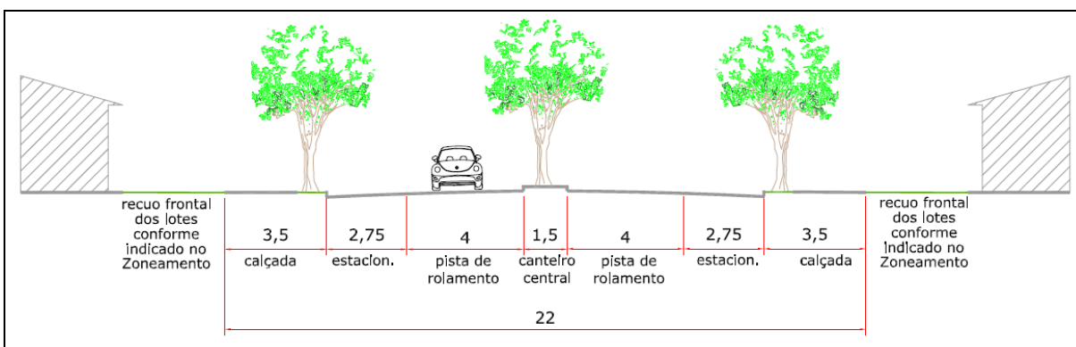
Figura 2 – Via Arterial Urbana. Fonte: MB Consultoria.
