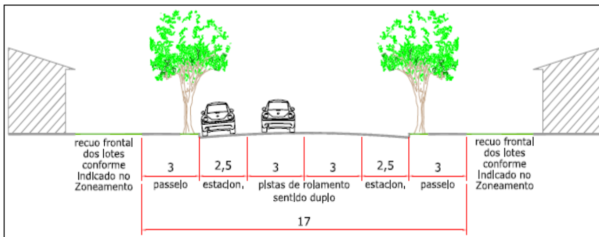
Figura 3 – Via Coletora. Fonte: MB Consultoria.
